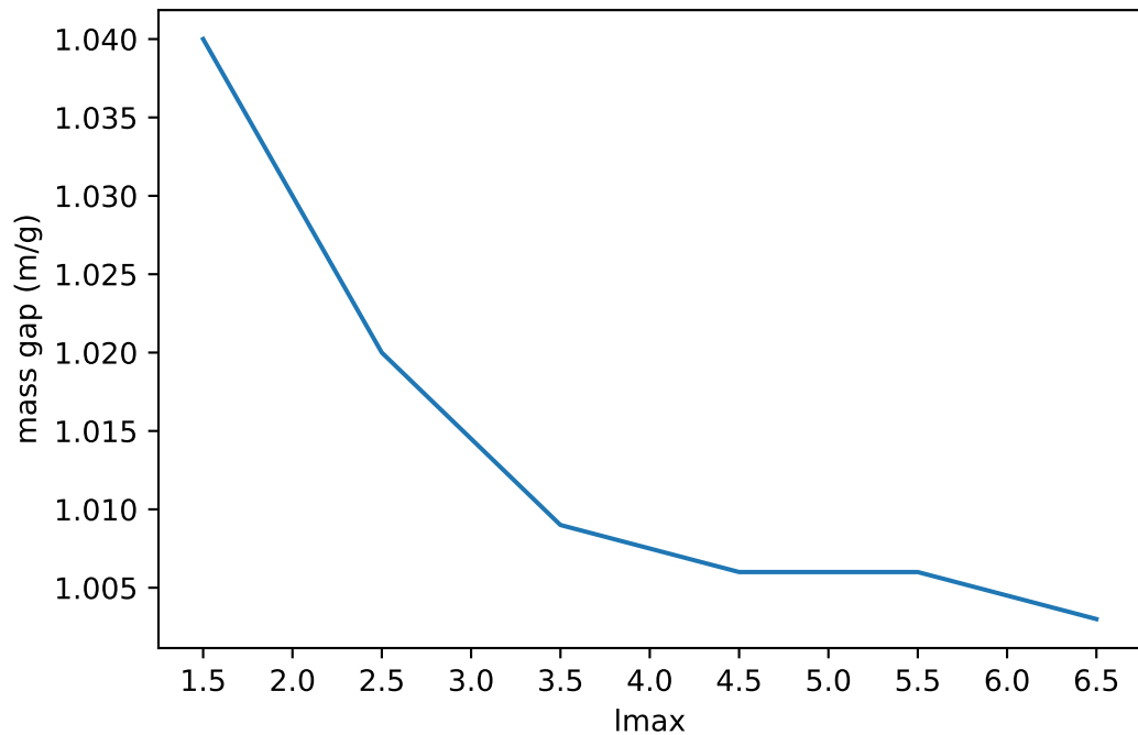
g=1, L=2\pi , antiperiodic case
