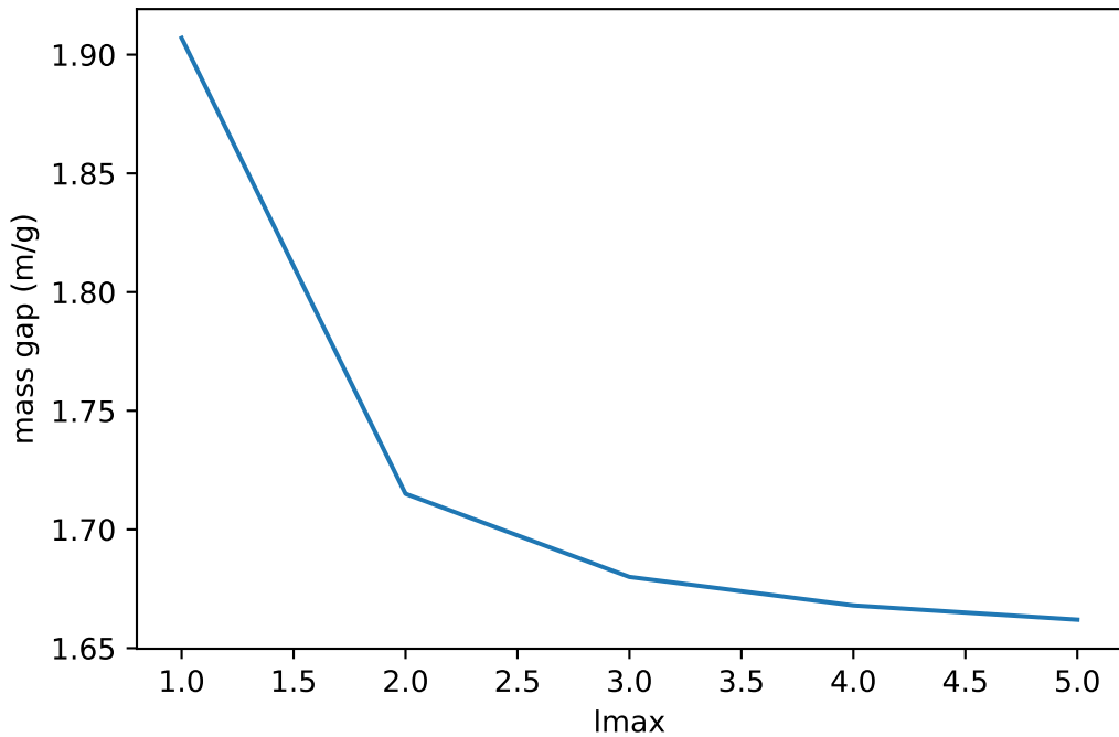
g=1, L=2\pi , periodic case
